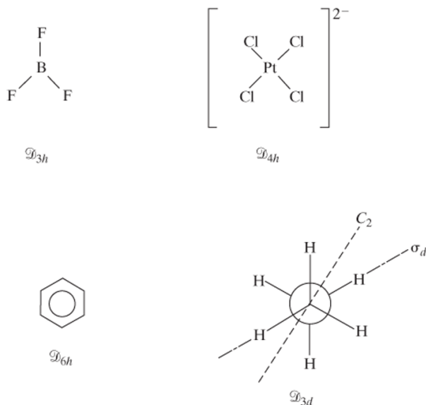
图 12.13: 具有一根 C_n 轴和 n 个 C_2 轴的分子。
