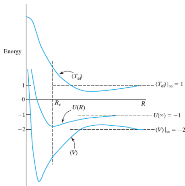
图 14.1: 双原子分子平均势能与动能的变化。能量单位取分离原子间的电子动能。
