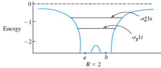
图 14.3: \text{H}_2^+ 分子在中等核间距条件下, 沿核间轴方向电子运动的势能。
