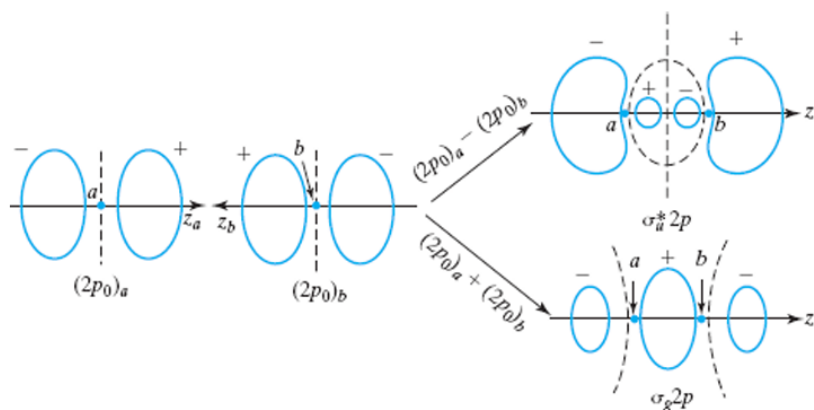
由 2p_z 原子轨道形成 \sigma_g 2p 和 \sigma_u^* 2p 分子轨道示意图。虚线表示节面。等高线上的符号表示波函数的符号。等高线关于图 13.11: z 轴对称。(由于 2s - 2p 轨道之间存在显著的杂化作用, 这些等高线并非真实分子轨道形状的准确表示。如需准确的等高线, 请参阅图 13.20。)
