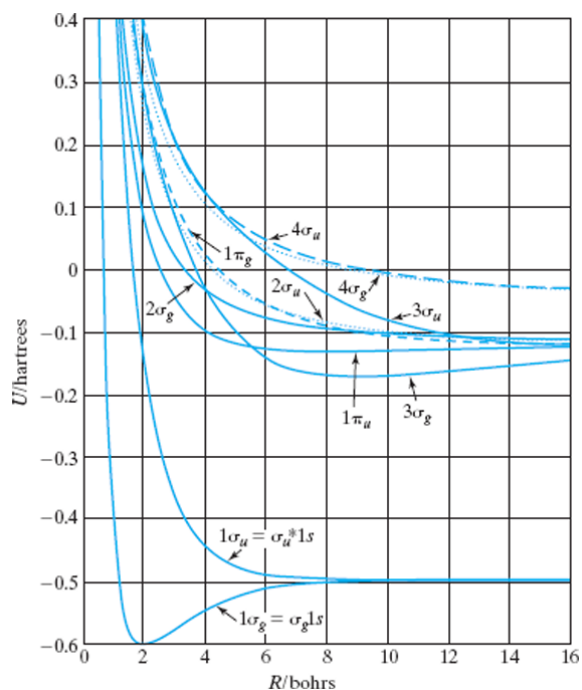
几个 H_2^+ 电子态的 U(R) 曲线。虚线用于帮助区分间隔较近的能级。在本图的尺度上无法观察到第一激发电子能级曲线在 12.5 bohrs 处的一个微小谷值，其势阱深度为 0.00006 hartrees。
