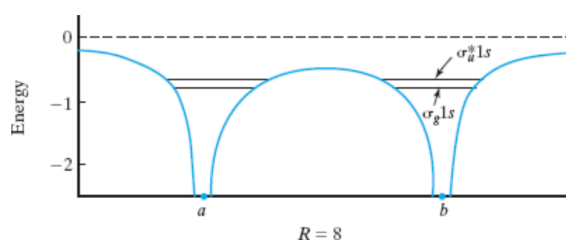
图 14.2: \text{H}_2^+ 分子在较大核间距条件下, 沿核间轴方向电子运动的势能。采用原子单位制。
